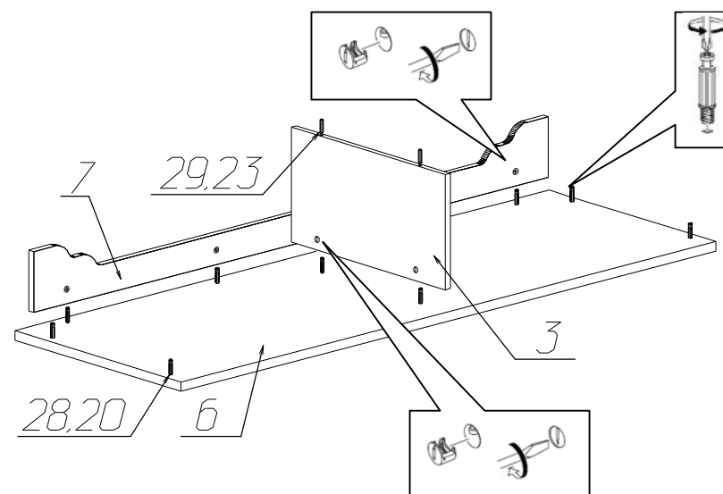
Инструкция по сборке шкафа № 668
